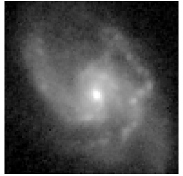
NEXUS F200W
