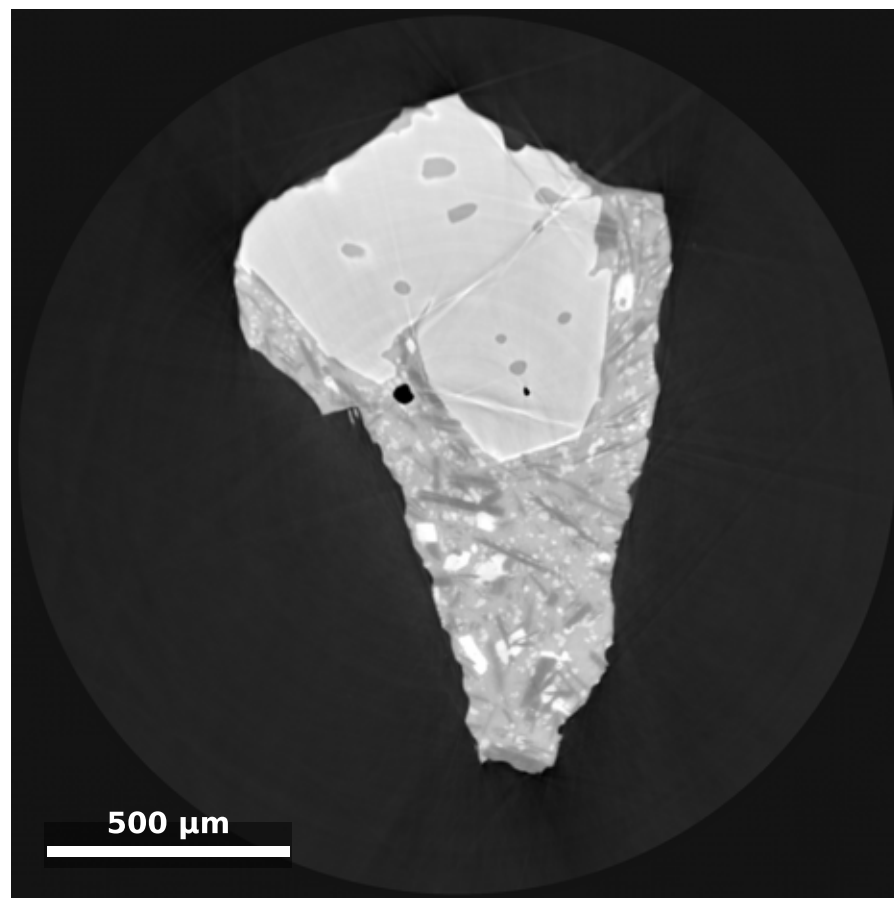
(d) Svartsengi March-May 2024 - Olivine
