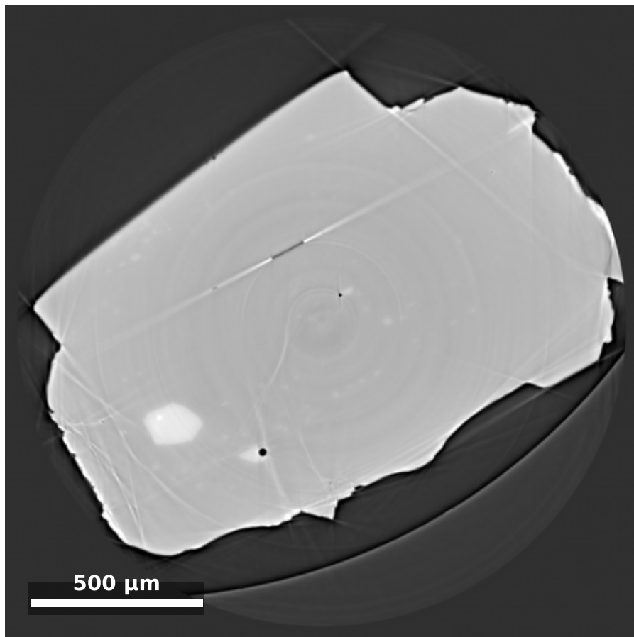
(a) Fagradalsfjall 2023 - Plagioclase
