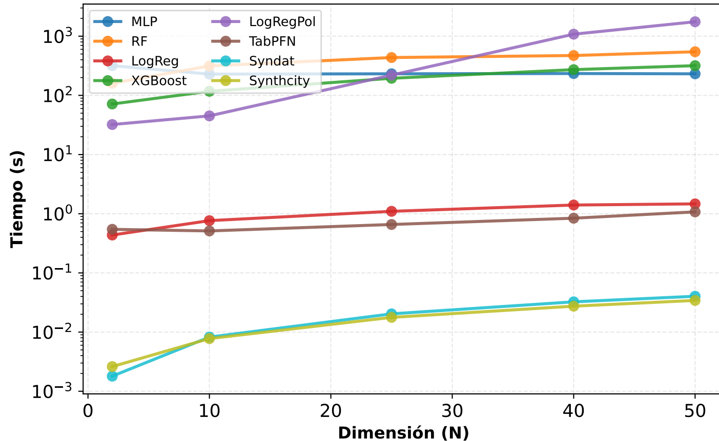
UC7: Tiempo de entrenamiento vs dimensión
