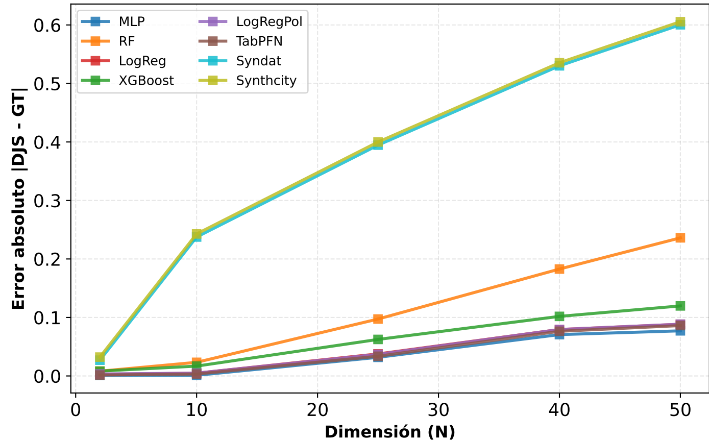
UC7: Error de estimación vs dimensión
