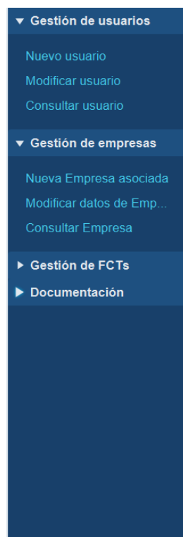
Imagen 10. Menú Administrador
