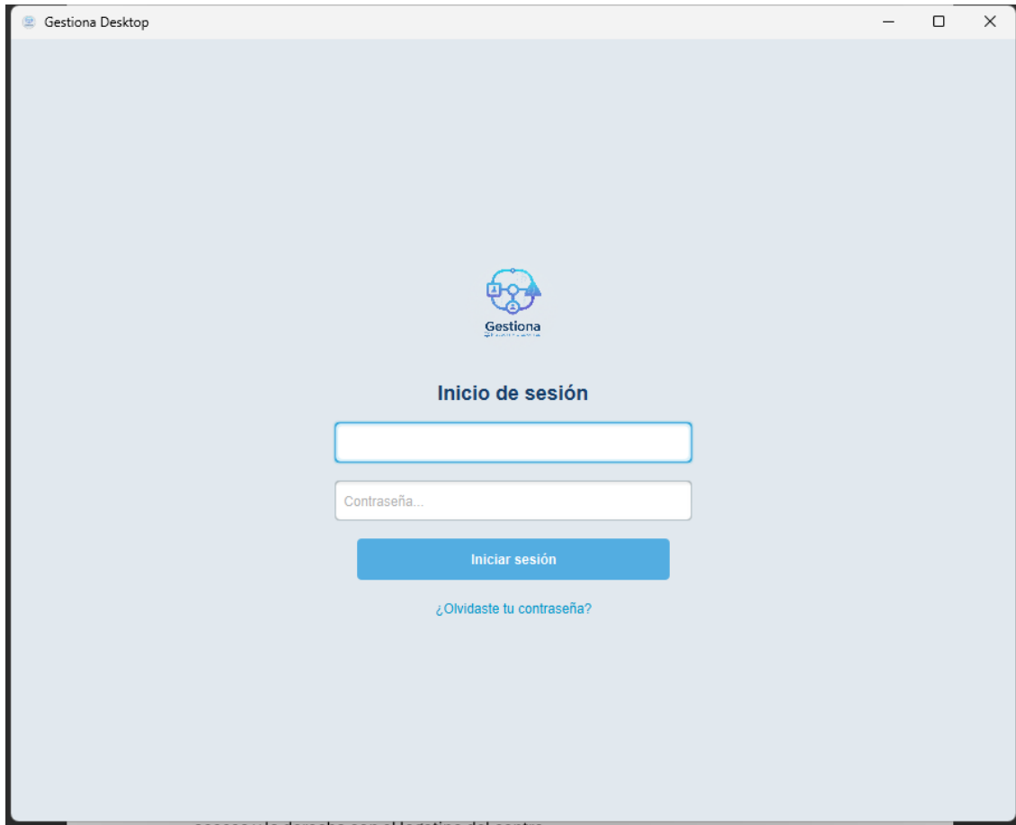
Imagen 28. pantalla Login
