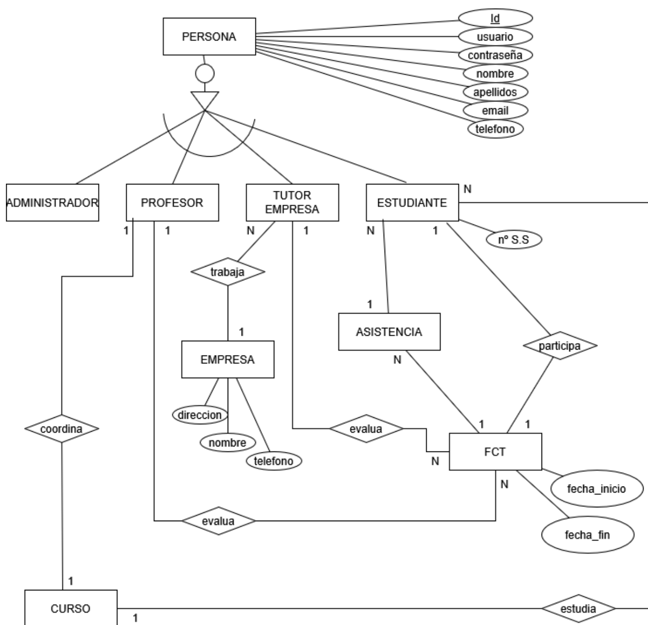
Figura 2. Diagrama Entidad/Relación
