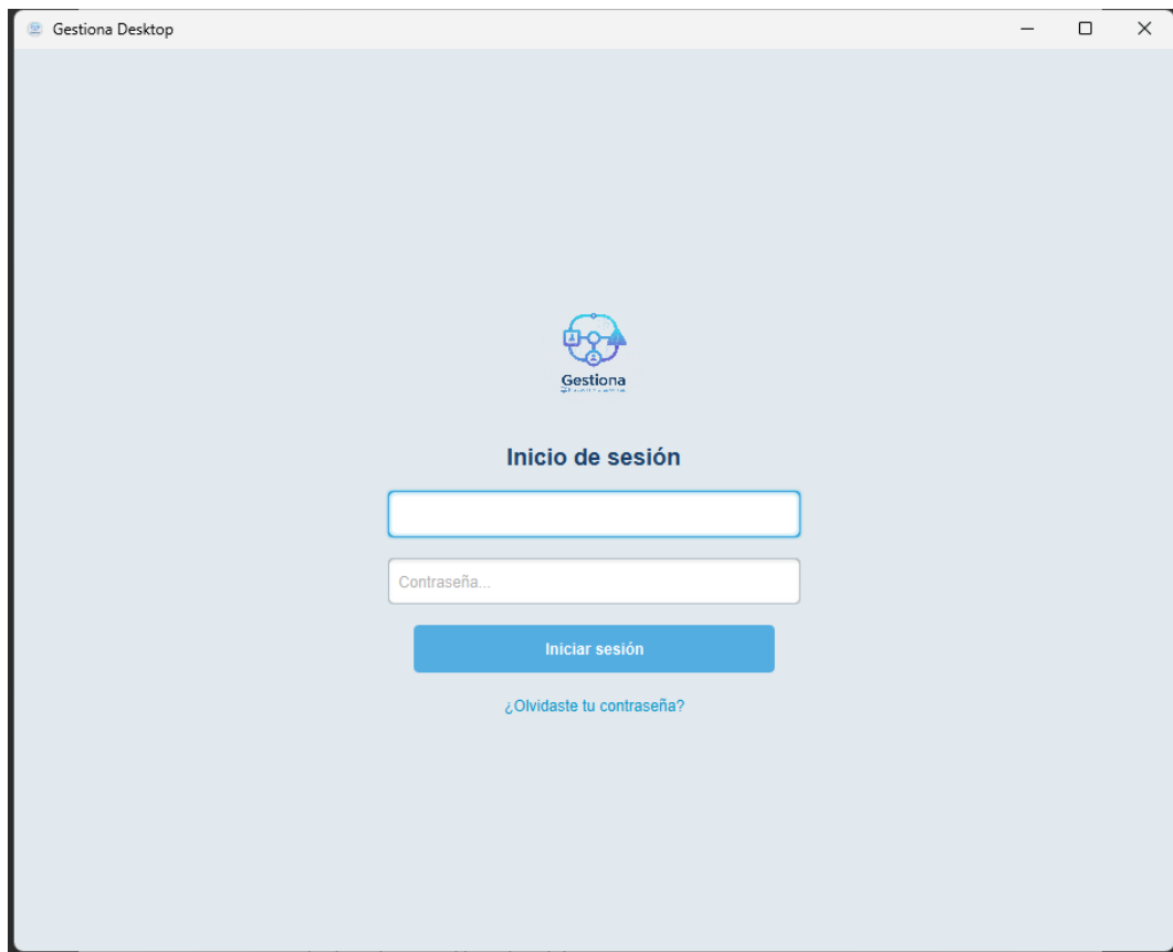
Imagen 27. Pantalla Login
