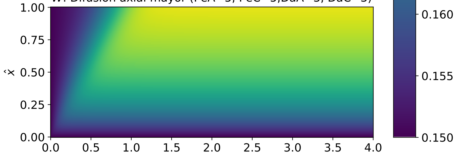
\hat{W} : Difusión axial mayor (PeA=5, PeC=5, DaA=3, DaC=3)
