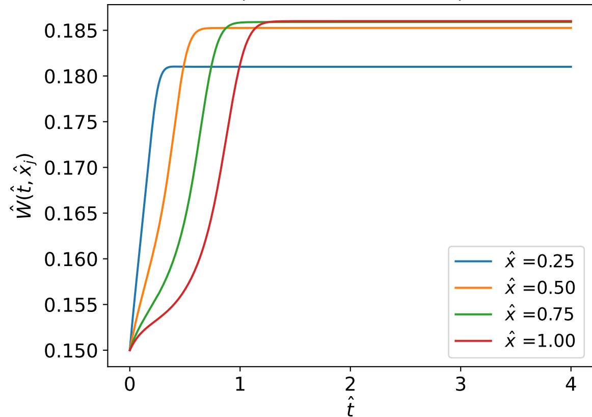
Evolución temporal de W - Caso: Acoplamiento alto
