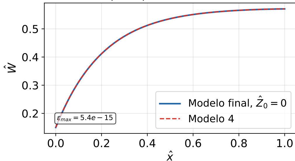
Canal capilar: perfil estacionario ( \hat{t} = 4 )
