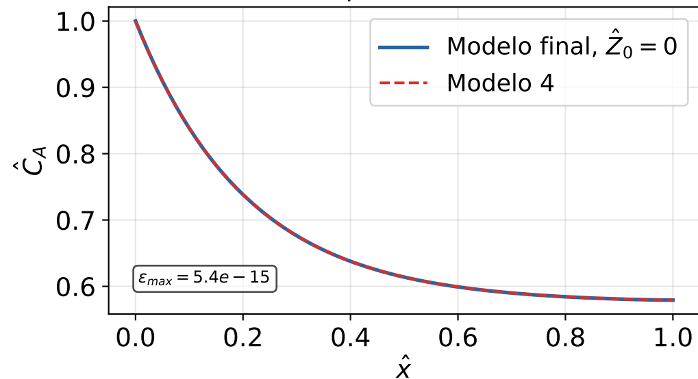
Canal alveolar: perfil estacionario ( \hat{t} = 4 )
