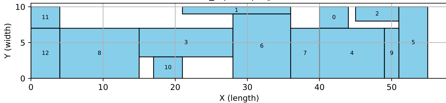
13_2 | tres | bigm
