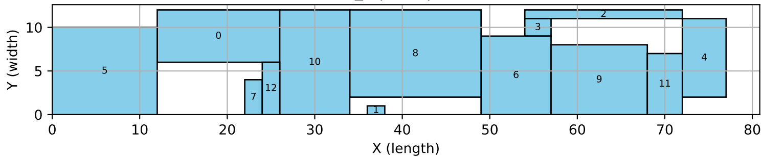
13_3 | tres | bigm
