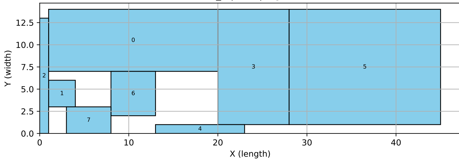
8_6 | tres | bigm
