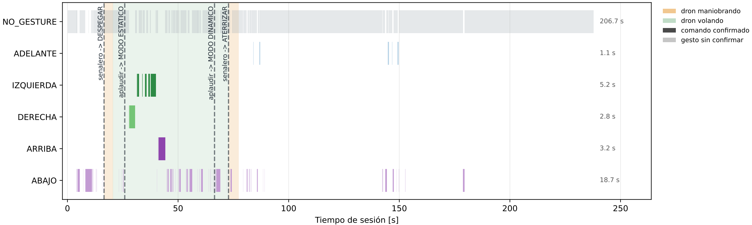
control_camara_dron1 · sesion_150127 · 2026-09-17 Comandos atendidos por el controlador en el tiempo (238 s, 5086 frames)
