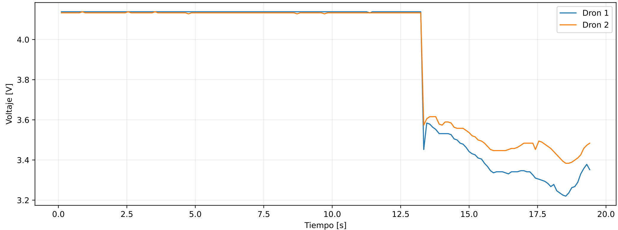
Voltaje de batería bajo carga
