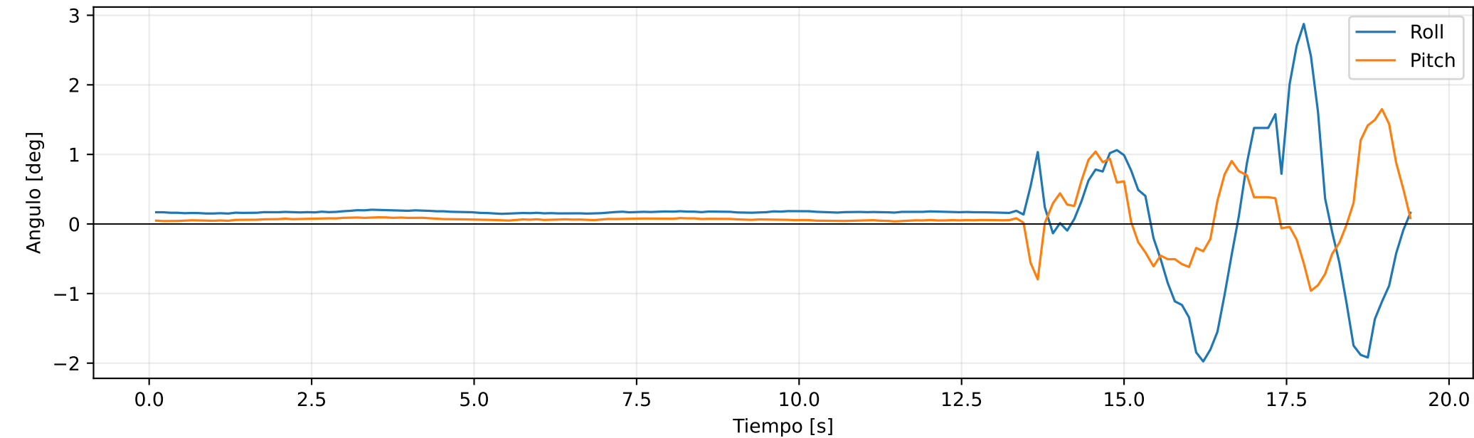
Dron 2: actitud
