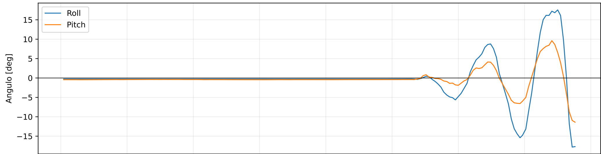
Dron 1: actitud
