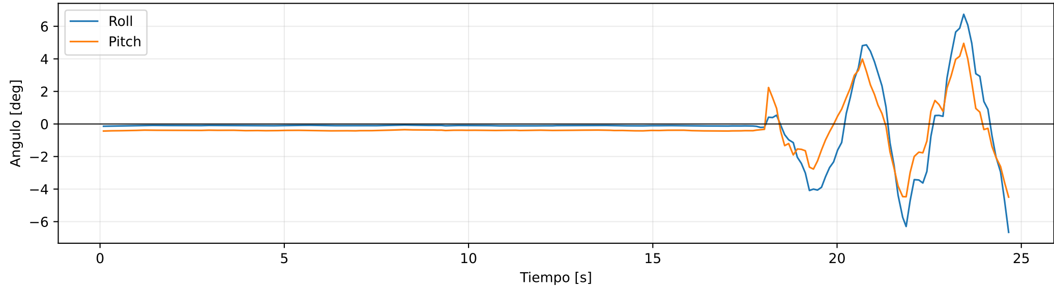
Dron 1: actitud
