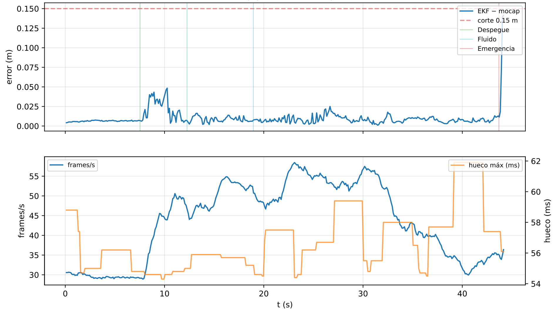
Error EKF-mocap y calidad del flujo del Robotat
