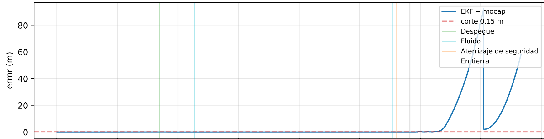
Error EKF-mocap y calidad del flujo del Robotat
