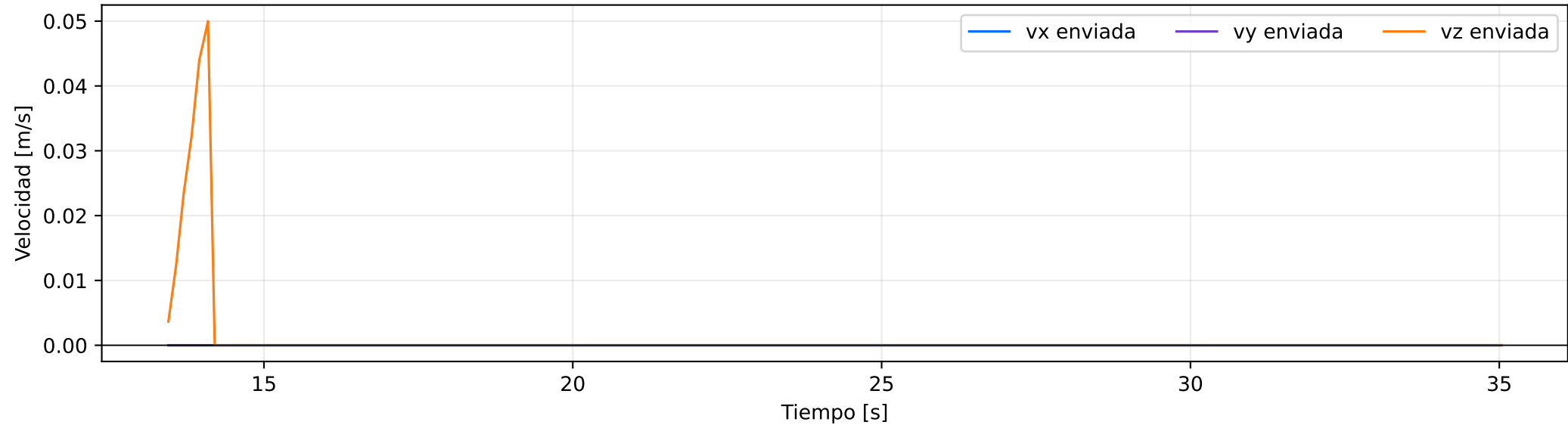
Dron 1: comandos de velocidad del lazo externo
