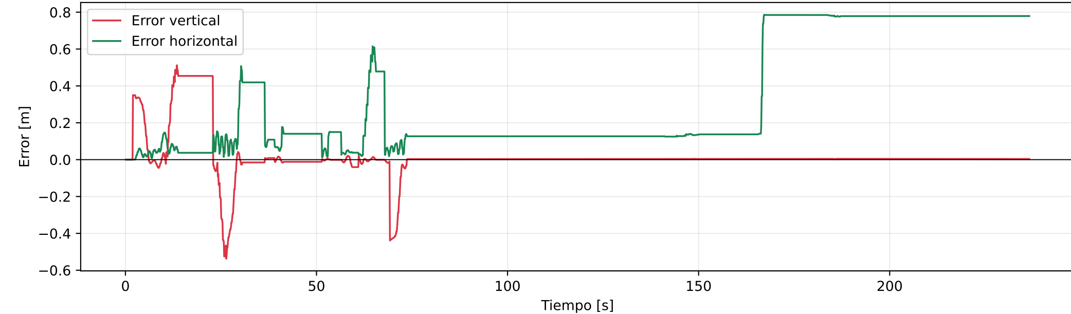
Dron 2: error respecto al objetivo
