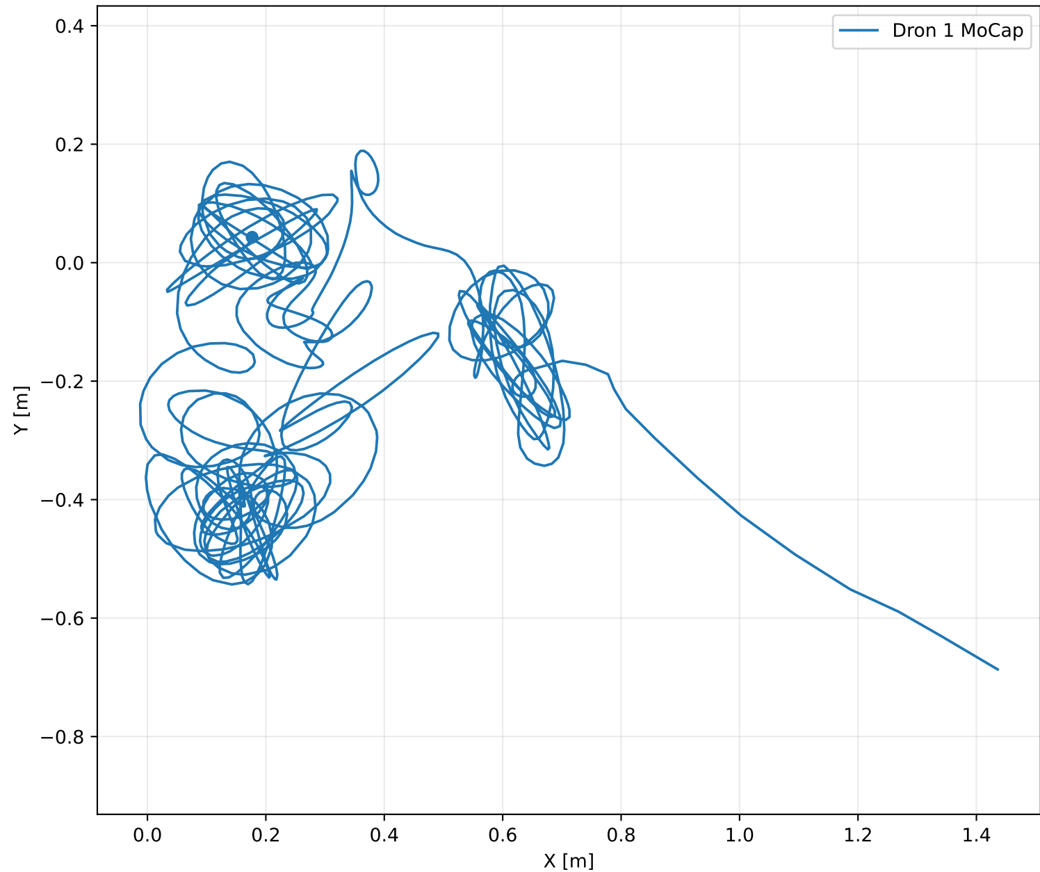
Trayectoria horizontal registrada
