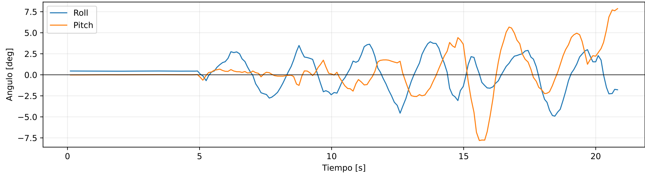
Dron 2: actitud
