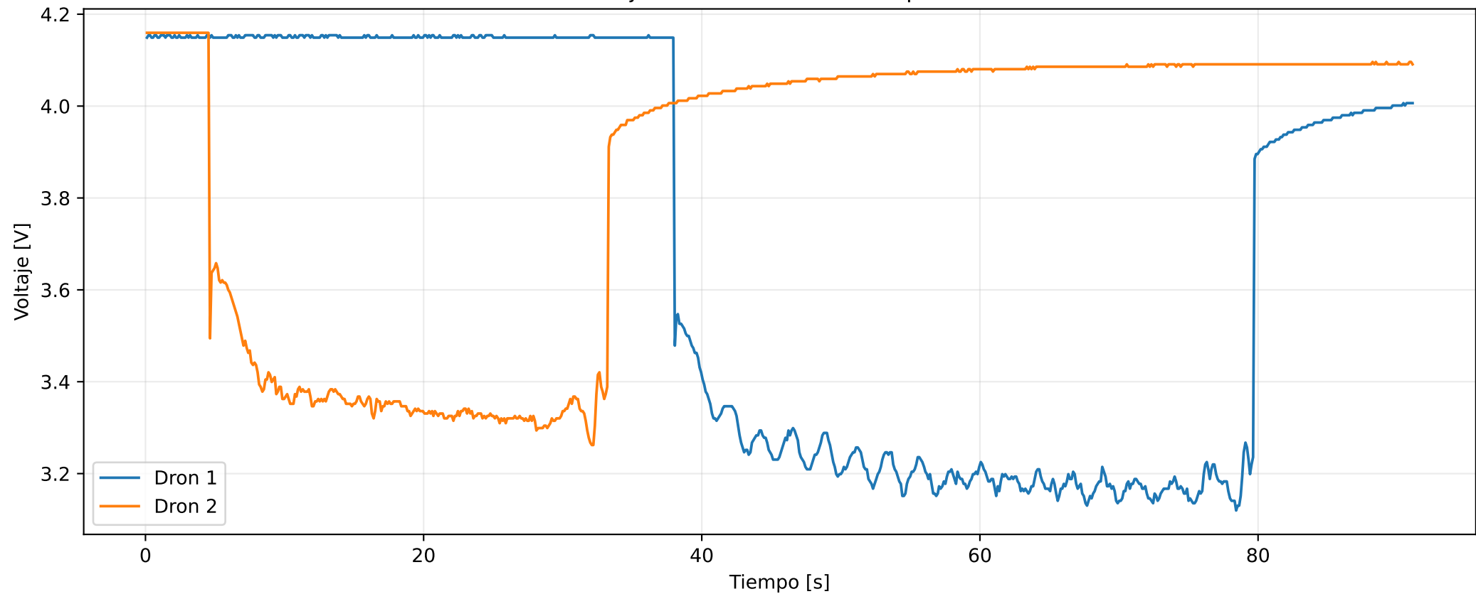
Voltaje de batería durante la prueba
