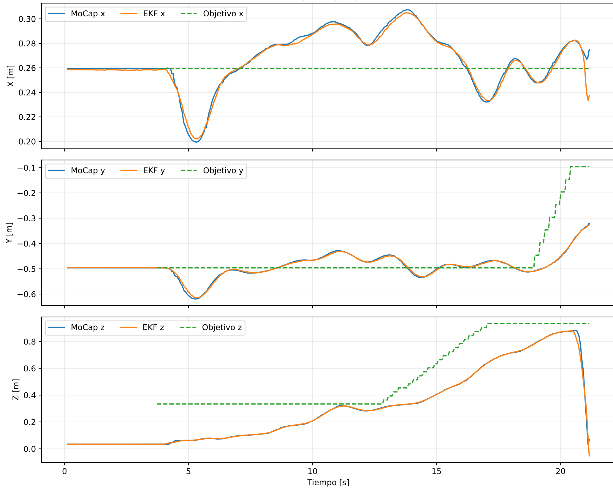
MoCap, EKF y objetivo
