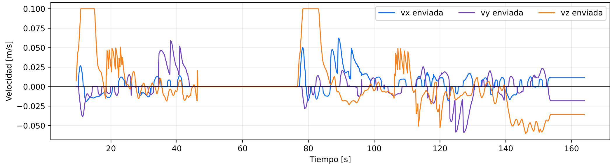
Dron 2: comandos de velocidad del lazo externo
