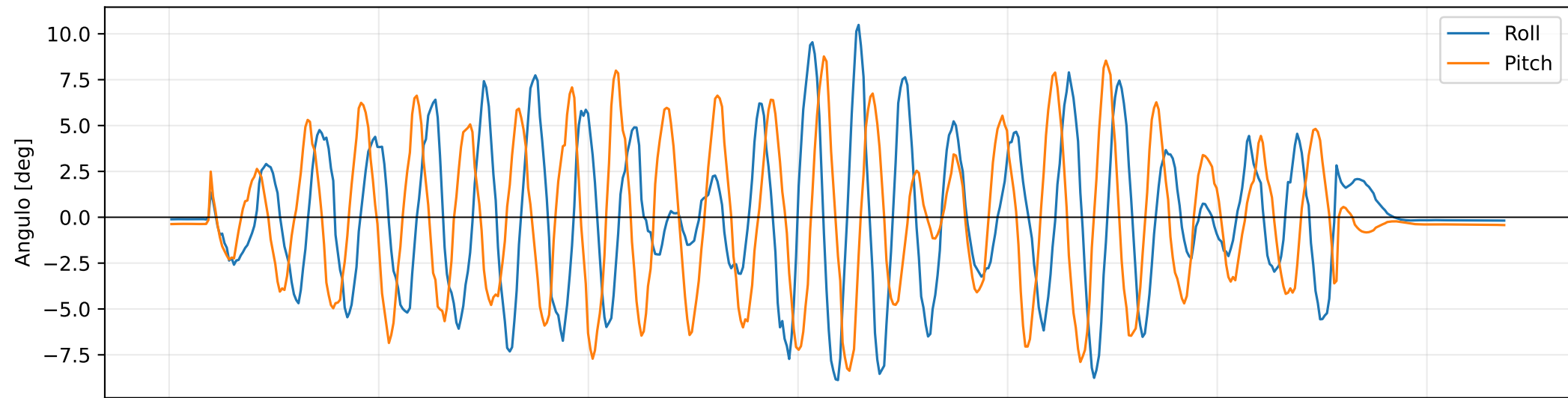
Dron 1: actitud
