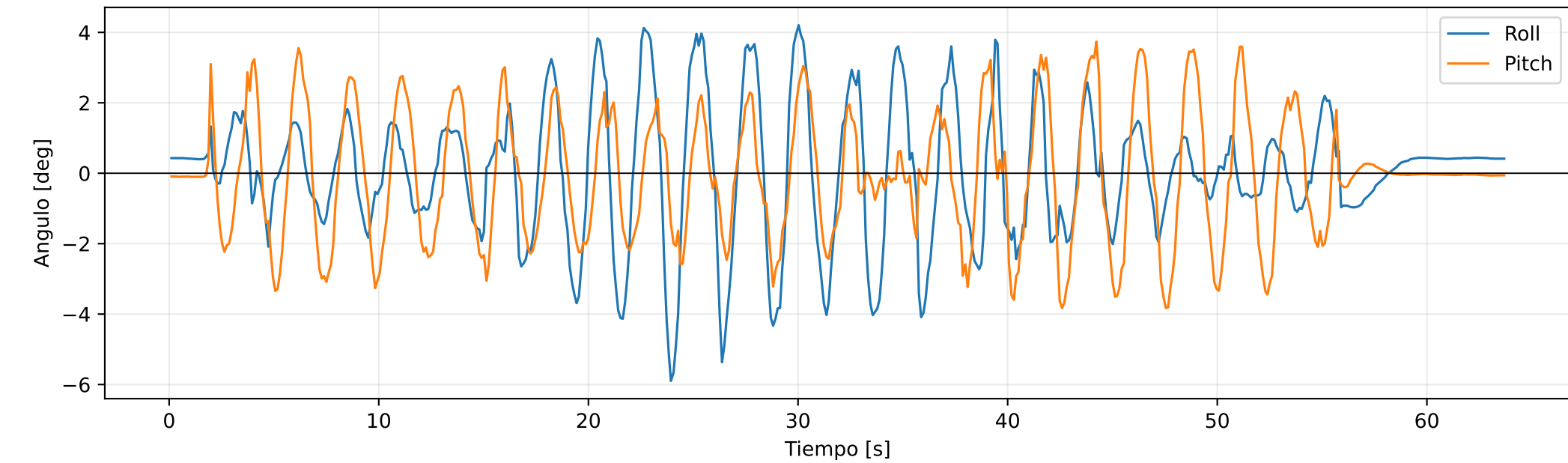
Dron 2: actitud
