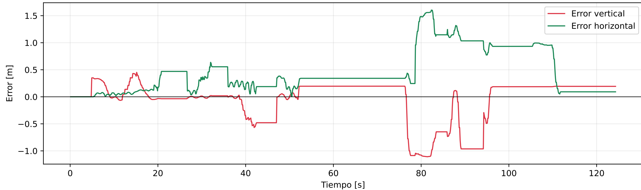
Dron 2: error respecto al objetivo
