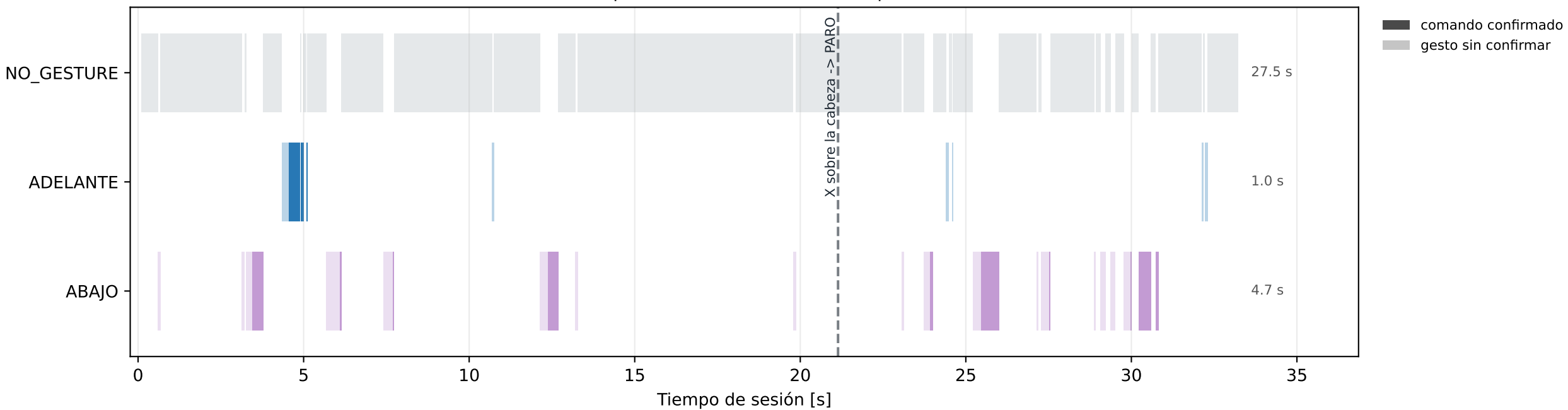
control_camara_dron1 · sesion_174620 · 2026-09-18 Comandos atendidos por el controlador en el tiempo (33 s, 713 frames)
