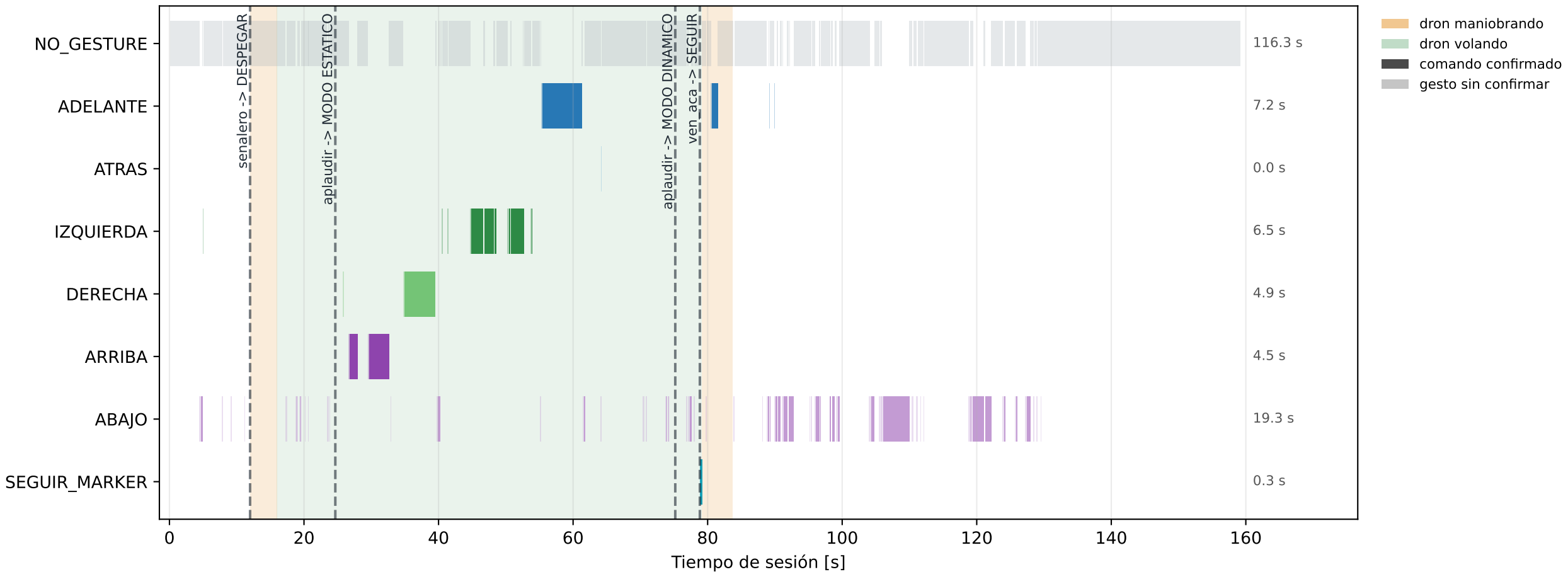
control_camara_dron1 · sesion_175102 · 2026-09-18 Comandos atendidos por el controlador en el tiempo (159 s, 3791 frames)
