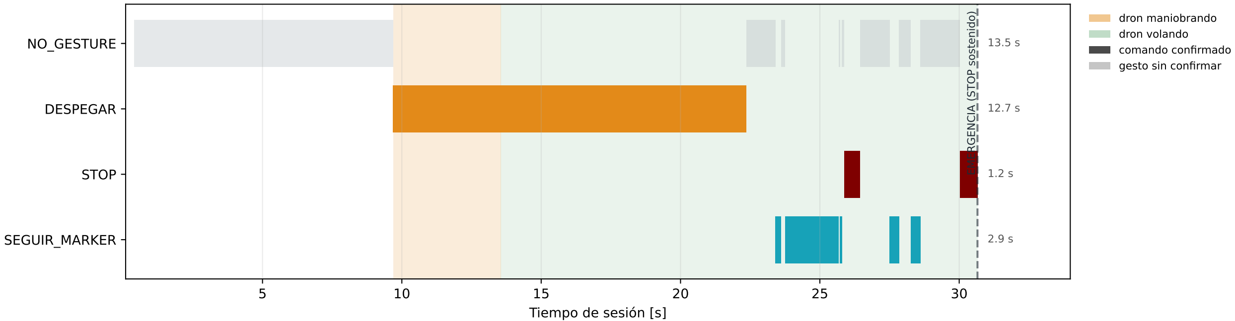
control_camara_dron1 · sesion_230213 · 2026-09-19 Comandos atendidos por el controlador en el tiempo (30 s, 908 frames)
