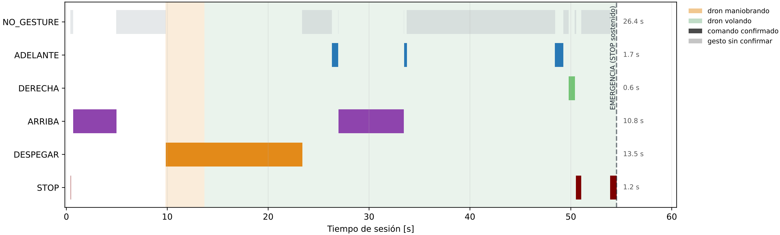
control_camara_dron1 · sesion_230314 · 2026-09-19 Comandos atendidos por el controlador en el tiempo (54 s, 1624 frames)
