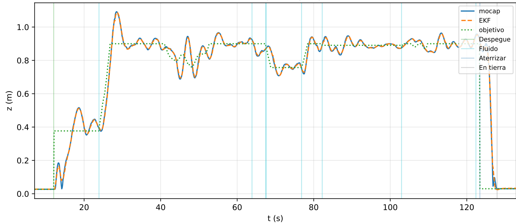
Altura: mocap, EKF y objetivo
