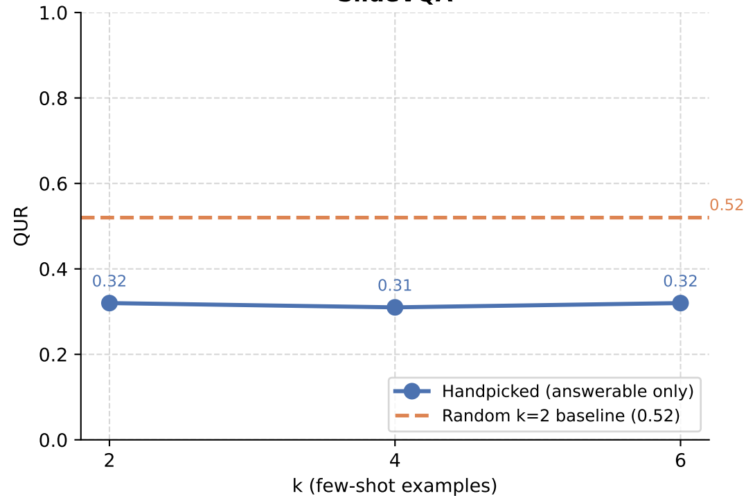
SlideVQA
