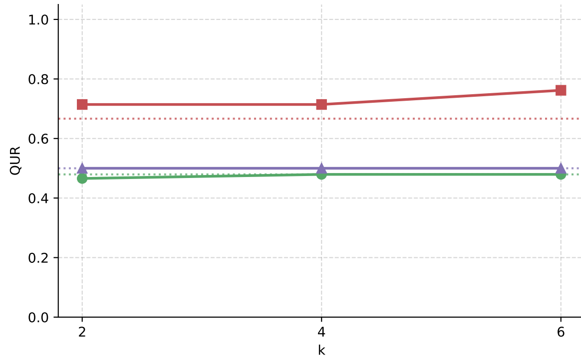
SlideVQA
