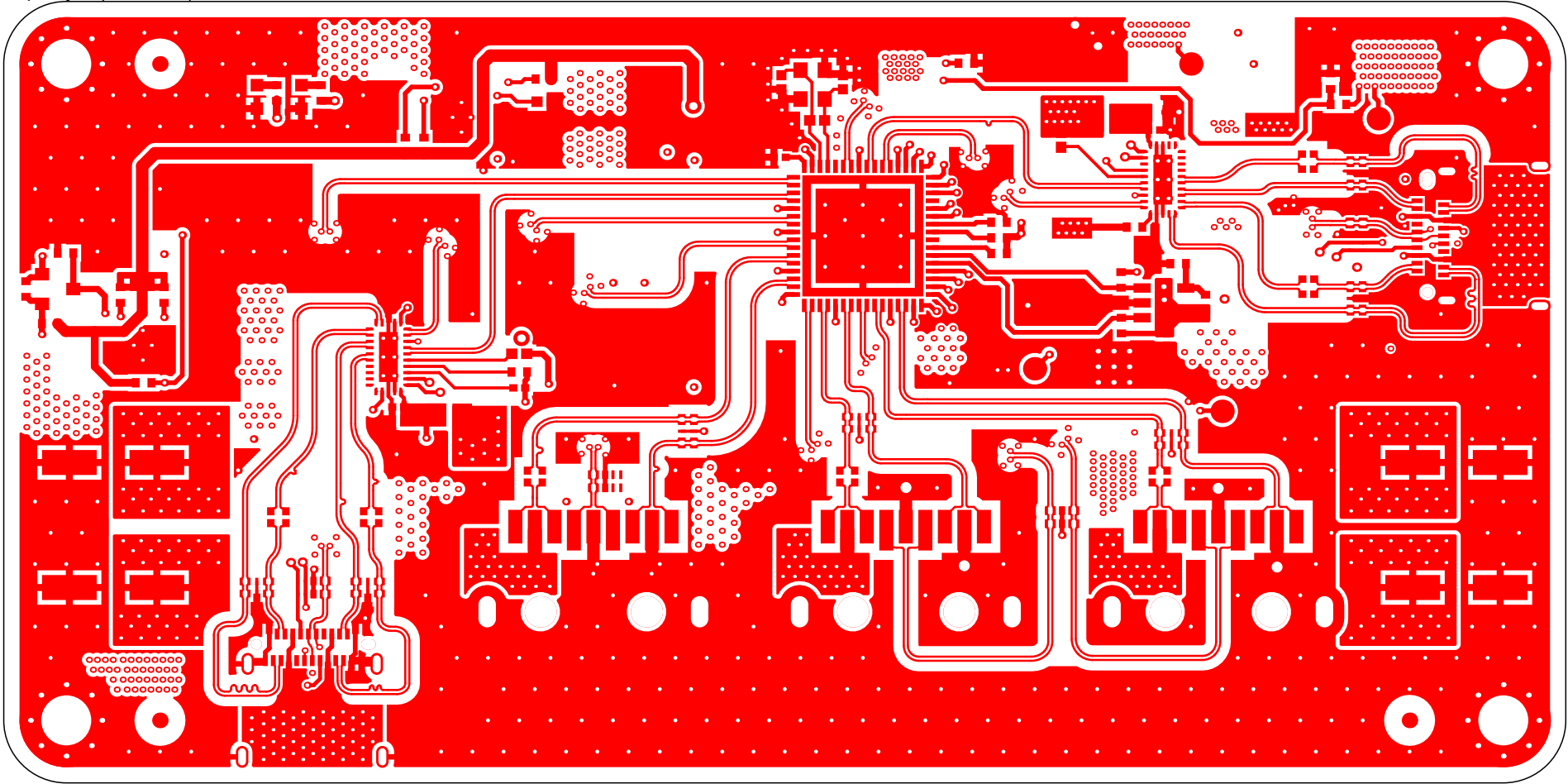
Top Layer (Scale 5:2)
