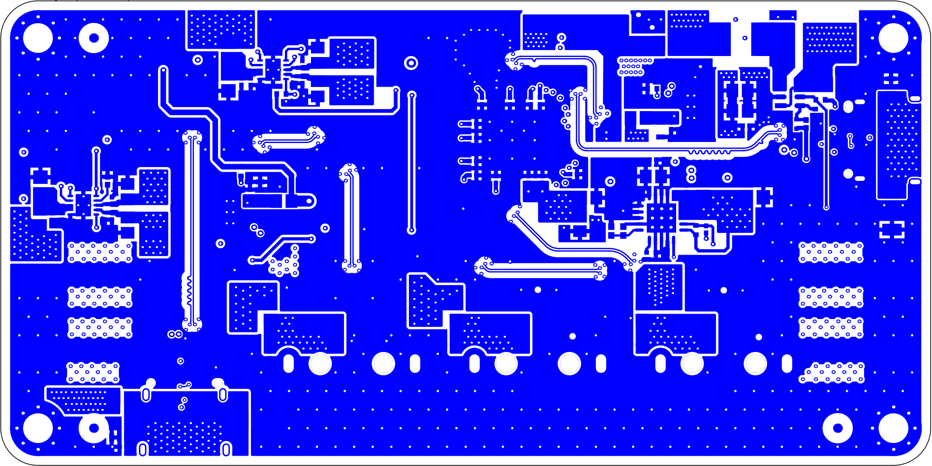
Bottom Layer (Scale 5:2)
