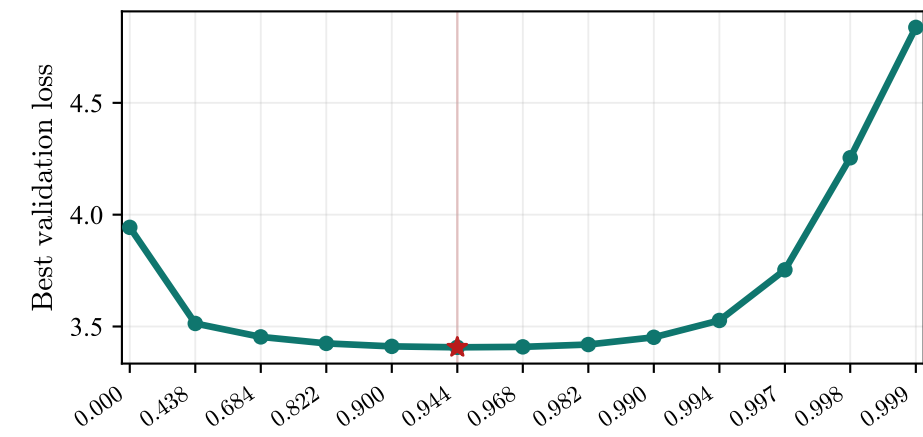
Llama60M on C4
