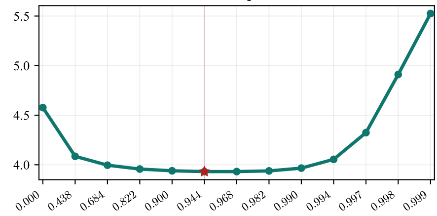
Llama60M on SlimPajama-6B
