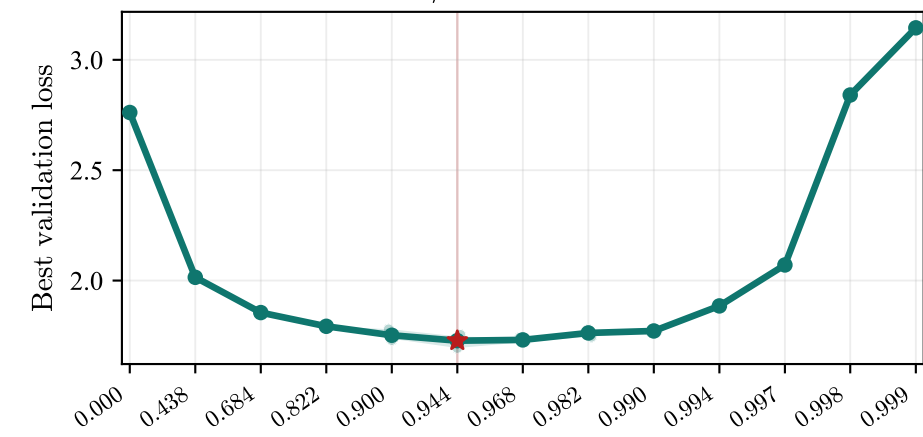
NanoGPT on WikiText-103
