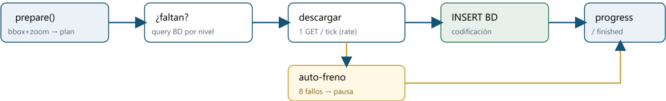
Figura 3 — Flujo de TileFiller : estima, descarga a ritmo, inserta con la codificación de la base y avisa; si hay muchos fallos seguidos, pausa y reanuda.
