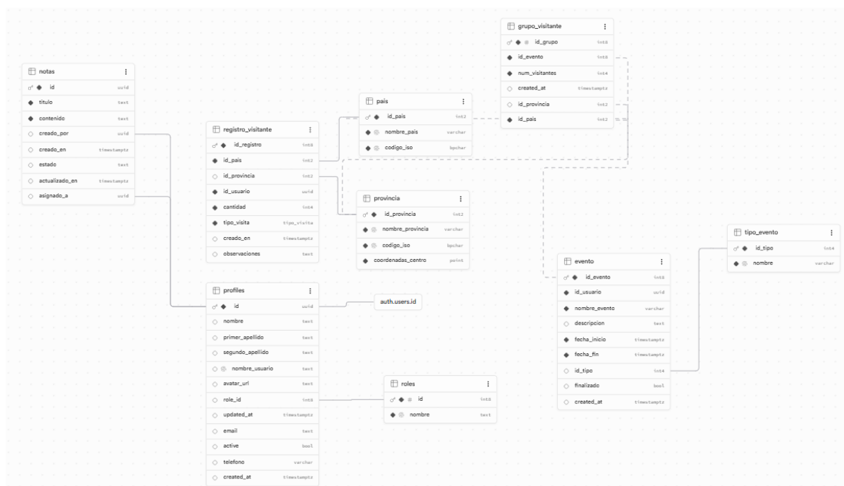
Figura 5.b — Diagrama de la base de datos de Visimap de Supabase
