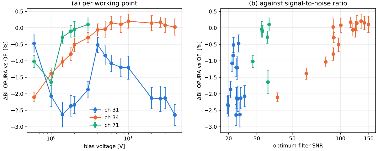
Figura 2: \Delta BI di OPURA rispetto all’algoritmo con i filtri, per i punti con tutti i 50 semi. Barre: larghezza della distribuzione dei \Delta BI sui semi. (a) In funzione della tensione di polarizzazione. (b) In funzione del rapporto segnale/rumore del filtro ottimo: il guadagno sta tutto dove l’SNR è basso.
