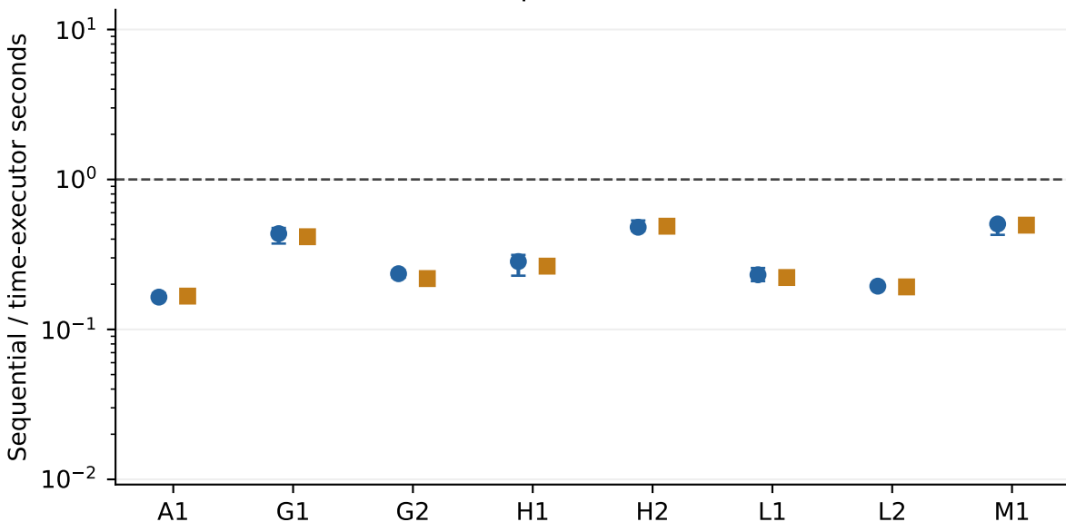
CUDA · quasi-DEER / MALA
