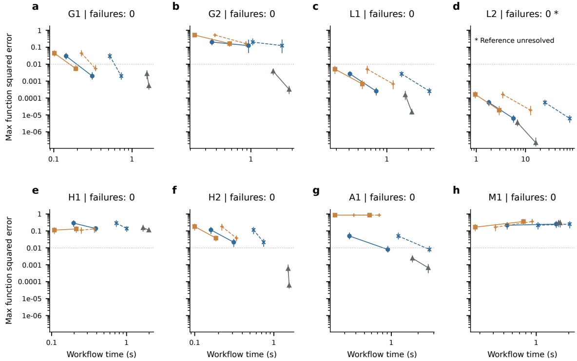
图 S2: 固定采样计划的误差—成本关系。横轴为成功输出条件下的 workflow 时间中位数, 全部尝试和失败成本另表保存。每条线连接同一指定工作流的两个预算点, 不表示中间预算已被测量。蓝色为 MALA、橙色为 RWM、灰色为 NUTS; 实线/圆或方形为顺序 MH, 虚线/叉号为相应时间执行器, 三角形为 NUTS。误差取预声明函数中最大的重复平均平方误差; L1/L2 为有限参考平方差。线段区间为逐点 95% 重复重采样区间, 有限参考的共同误差敏感性另行传播; 传播采用正态对角协方差工作假设, 非同时保证。星号表示参考精度未确定, 该面板仅供探索性平方差比较。面板标题列出该模型全部正式任务中的输出失败数, 失败组的误差为条件结果。点虚线标出 0.01 作为预声明误差阈值。
