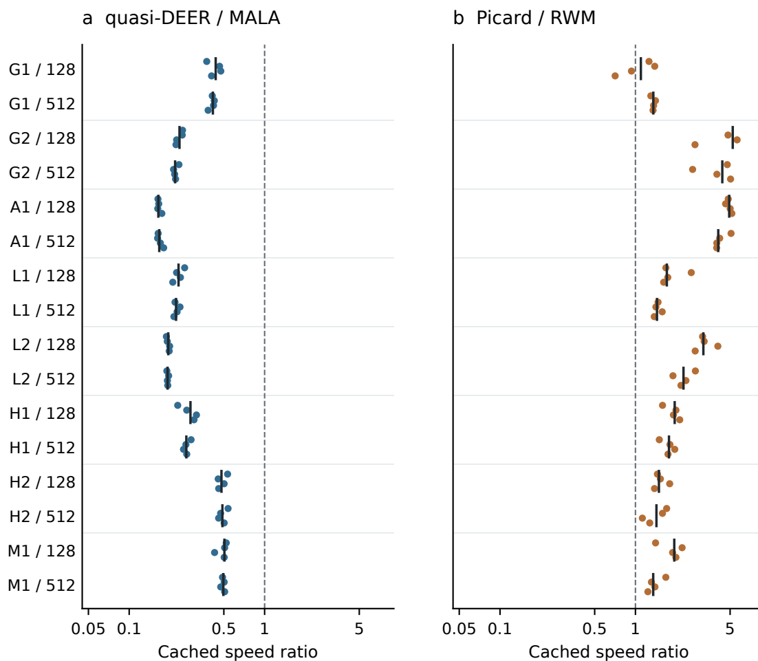
图 S6: 首轮 Windows CUDA 全部配对点, 每行四份原始输入; 黑线为中位数, 虚线为速度比 1。左为 quasi-DEER MALA, 右为 Picard RWM。该历史预算和配置不与紧凑研究混合。
