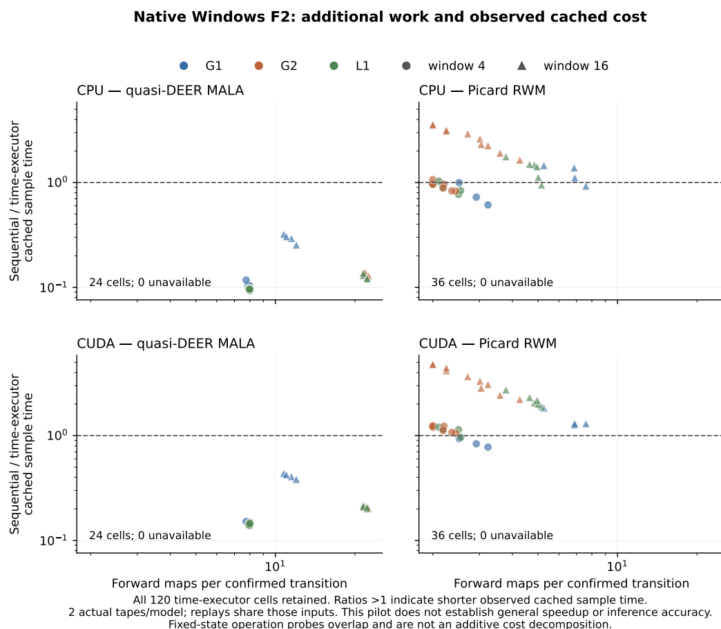
图 S5: Windows 机制测量中的重复求值与缓存成本。每点为一个配置与实际输入的组合, 共 120 点, 部分重叠; 颜色区分目标, 点形区分窗口。上下行为 CPU/CUDA, 左右列为 quasi-DEER/Picard。纵轴大于 1 表示指定缓存执行较短; 横轴包括拒绝自环。三次技术重放不扩充独立样本量, 图中没有推断精度或统计区间。操作探针存在重叠, 不用于构造可加的独占耗时分解。
