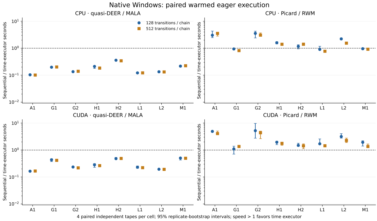
图 S4: 原生 Windows 配对执行结果; 每组 4 份独立数组, 误差线为重复层面 2000 次 bootstrap 的逐点 95% 区间, 不提供同时置信保证。CUDA Picard 的 16 组中位数大于 1, 其中 15 组区间下限大于 1。A1/RWM 的全部 32 次拟合均拒绝所有提议, 其速度仅反映自环执行, 不能解释为后验探索加速。quasi-DEER 的所有组中位速度比均小于 1; 全部负结果保留。
