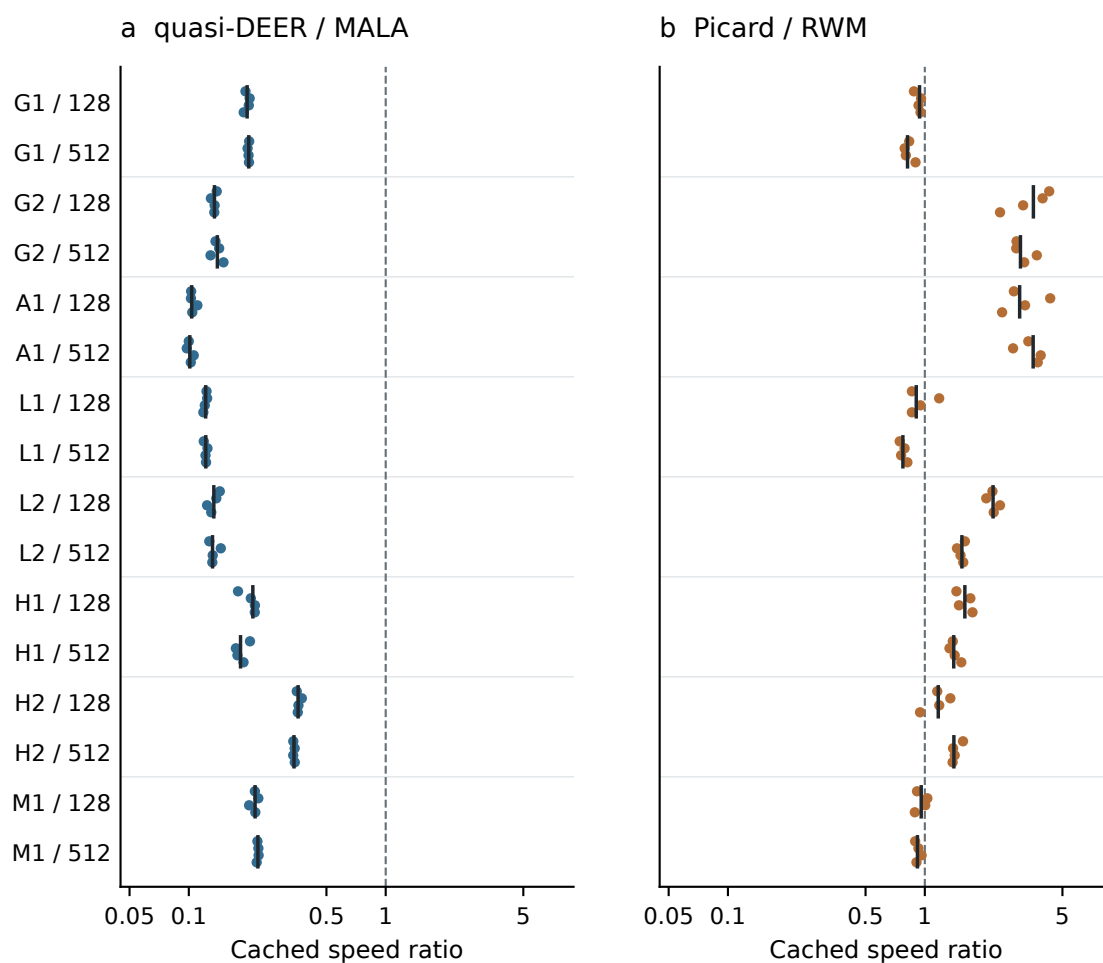
图 S7: 首轮 Windows CPU 全部配对输入的缓存速度比。四个点为每格四份实际数组; 黑色短线为中位数, 不作置信区间。两个面板依次对应 quasi-DEER MALA 与 Picard RWM。
