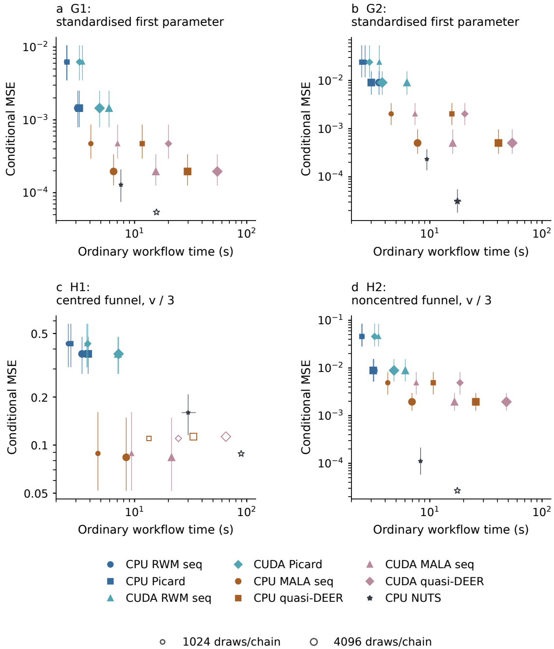
图 3: 已测预算上的函数误差与普通工作流耗时。事后为解释简单目标、白化后维度和漏斗参数化而选择 G1/G2 的标准化首参数均值及 H1/H2 的 v/3 ; 四面板均保留全部九工作流、两预算, 其他函数见完整结果附录图 R2–R45。点大小区分 1024/4096 预算, 横纵线为逐点 95% BCa 区间, 空心点表示区间未定。每点计划 24 份四链重复; G1/G2/H2 的 MH 均为 24 份, Pyro NUTS 分别为 24/7、24/24、24/7; H1 的 RWM 为 24/24, 顺序 MALA 为 24/23, quasi-DEER 为 17/11, NUTS 为 24/9。点为各自有效集合的描述, 共同集合上的损失比较另见完整附录。
