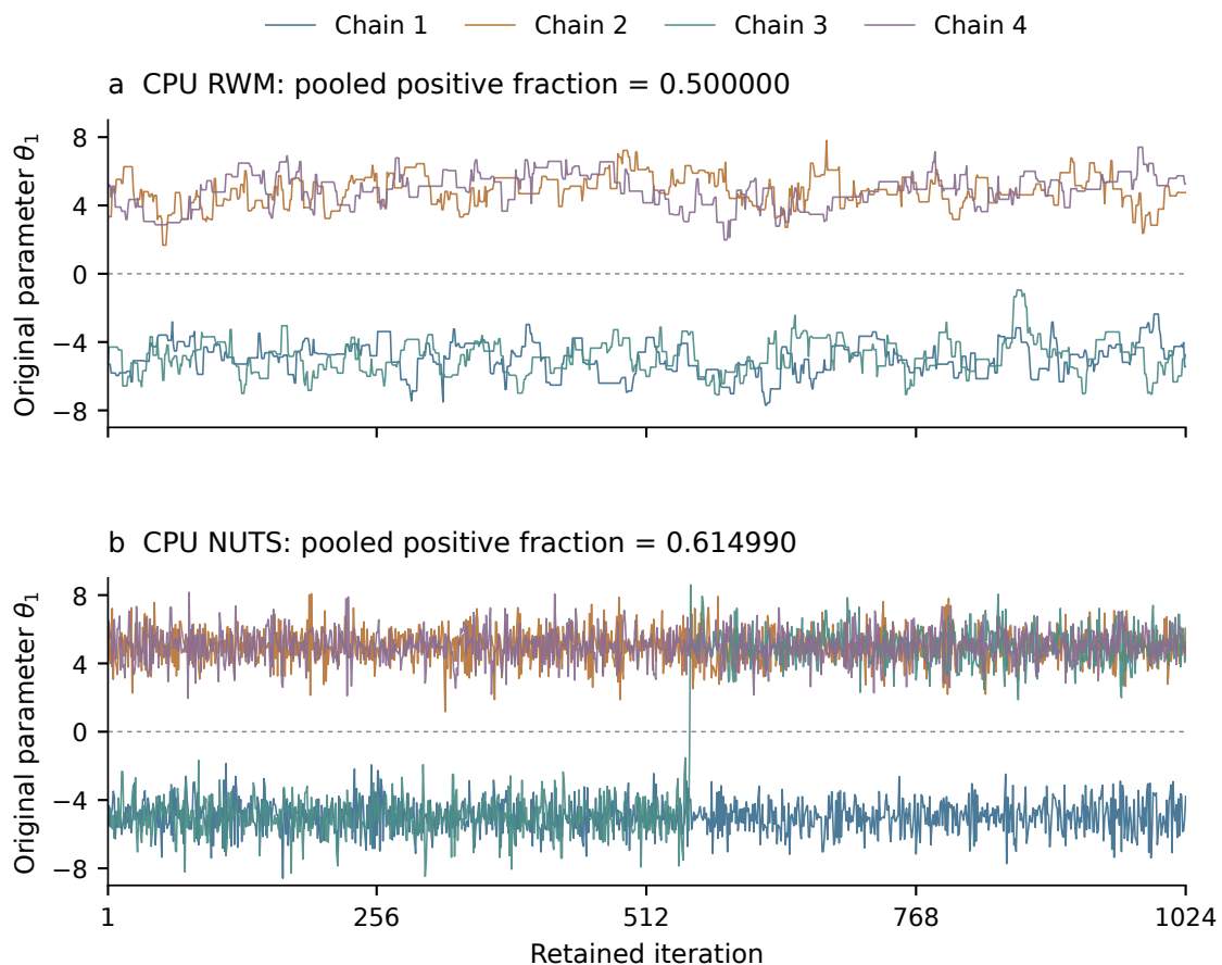
图 4: 双峰目标的保存路径。上图为 CPU 顺序 RWM, 下图为完整 M1 审查中唯一出现符号穿越的 CPU NUTS 拟合, 两者为同一原重复和 1024 步预算, 初值相同但随机机制不同。绘出四链全部保留状态; \theta_1 为原尺度上的第一参数。示例按上述事后规则选择, 不据两份拟合比较性能。
