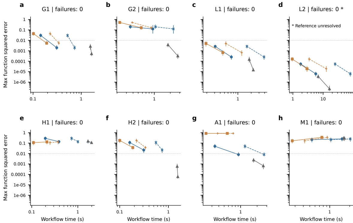
图 2: 固定采样计划的误差—成本关系。横轴为成功输出条件下的工作流时间中位数，全部尝试和失败成本另表保存。每条线连接同一指定工作流的两个预算点，不表示中间预算已被测量。蓝色为 MALA、橙色为 RWM、灰色为 NUTS；实线/圆或方形为顺序 MH，虚线/叉号为相应时间执行器，三角形为 NUTS。误差取预声明函数中最大的重复平均平方误差；L1/L2 为有限参考平方差。线段区间为逐点 95% 重复重采样区间，有限参考的共同误差敏感性另行传播；传播采用正态对角协方差工作假设，非同时保证。星号表示参考精度未确定，该面板仅供探索性平方差比较。面板标题列出该模型全部正式任务中的输出失败数，失败组的误差为条件结果。点虚线标出 0.01 作为预声明误差阈值。
