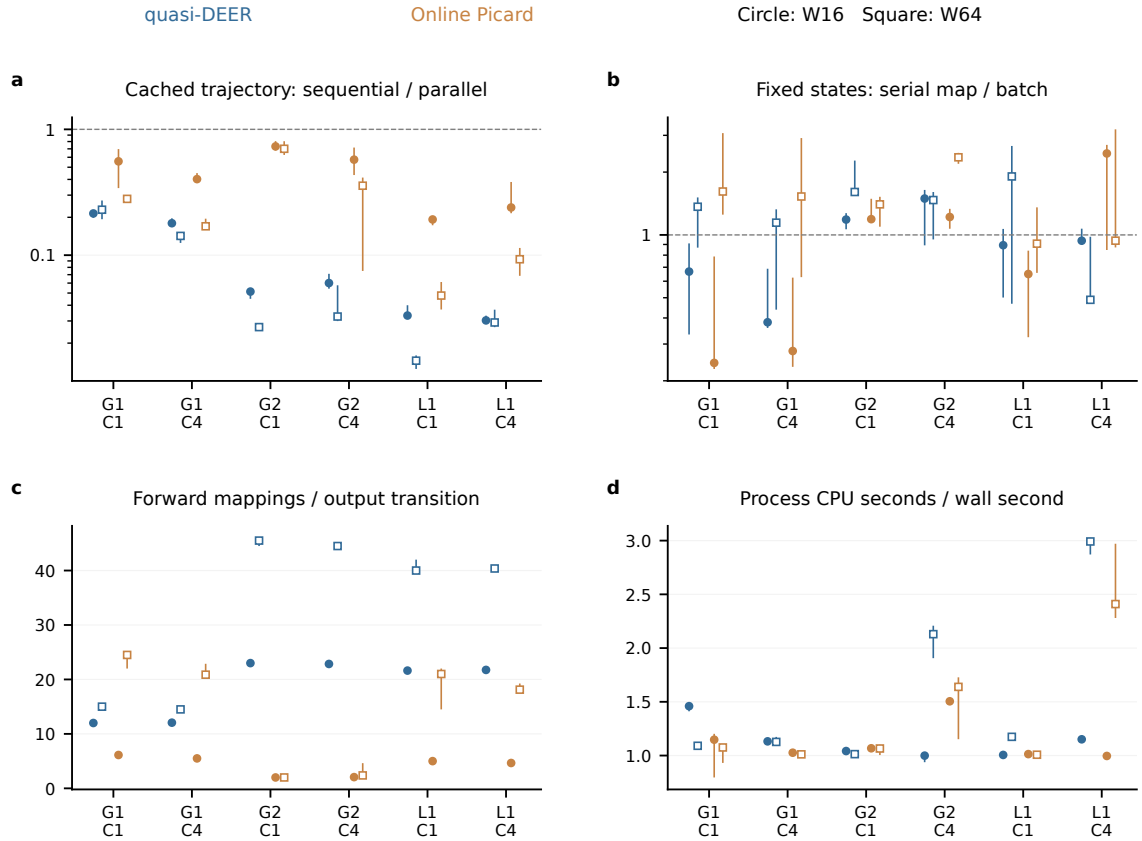
图 3: 新冻结的 72 项机制任务。每格 3 个实际随机数组, 符号为组中位数, 细线为最小至最大值; 技术计时重复不扩大样本量。蓝色为 quasi-DEER, 橙色为 Picard; 圆点为窗口 16, 方形为 64; 横轴 C 为链数。a: 缓存轨迹速度比, 1 以上才为加速。b: 固定状态批量吞吐比, 1 以上表示批处理有利, 但它不是轨迹加速。c: 每个输出转移的前向映射求值数, quasi-DEER 还另有 JVP; 拒绝自环计入转移。d: 进程 CPU 秒/墙钟秒, 表示观测消费量而非核数配置。
