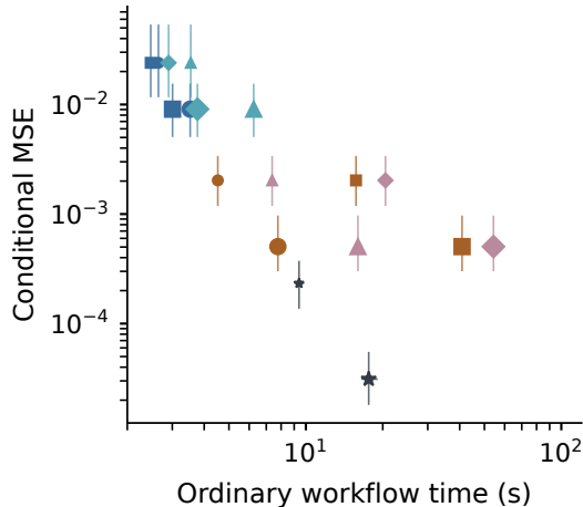
b G2: standardised first parameter
