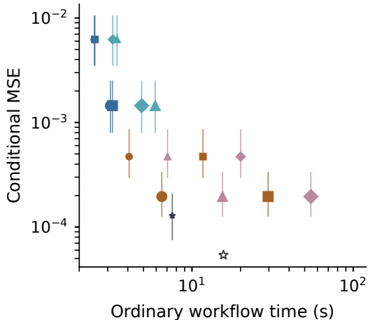
a G1: standardised first parameter
