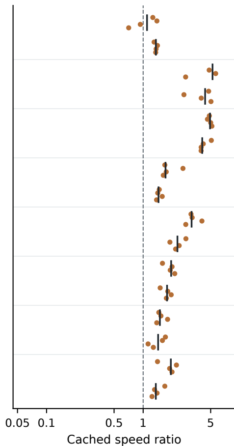
b Picard / RWM
