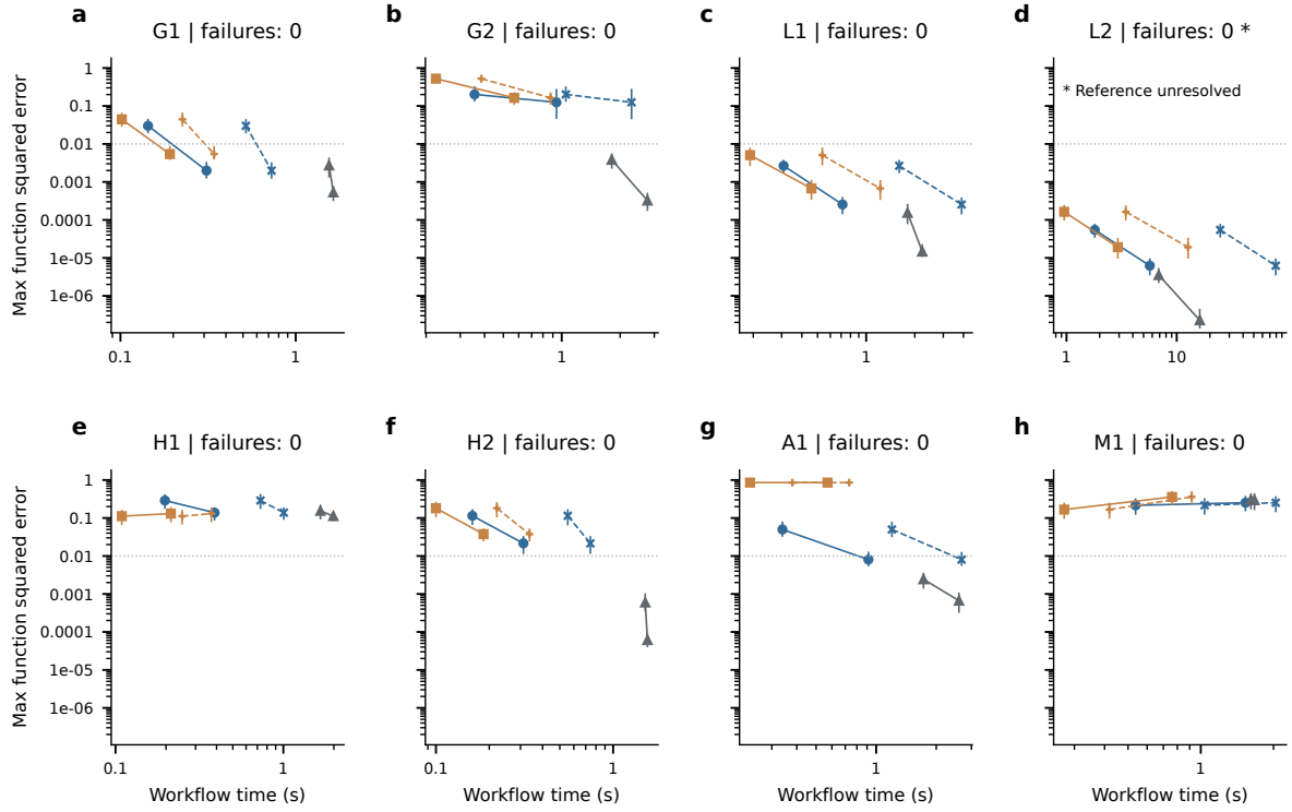
图 2: 固定采样计划的误差—成本关系。横轴为成功输出条件下的 workflow 时间中位数, 全部尝试和失败成本另表保存。每条线连接同一指定工作流的一个预算点, 不表示中间预算已被测量。蓝色为 MALA、橙色为 RWM、灰色为 NUTS; 实线/圆或方形为顺序 MH, 虚线/叉号为相应时间执行器, 三角形为 NUTS。误差取预声明函数中最大的重复平均平方误差; L1/L2 为有限参考平方差。线段区间为逐点 95% 重复重采样区间, 有限参考的共同误差敏感性另行传播; 传播采用正态对角协方差工作假设, 非同时保证。星号表示参考精度未确定, 该面板仅供探索性平方差比较。面板标题列出该模型全部正式任务中的输出失败数, 失败组的误差为条件结果。点虚线标出 0.01 作为预声明误差阈值。
