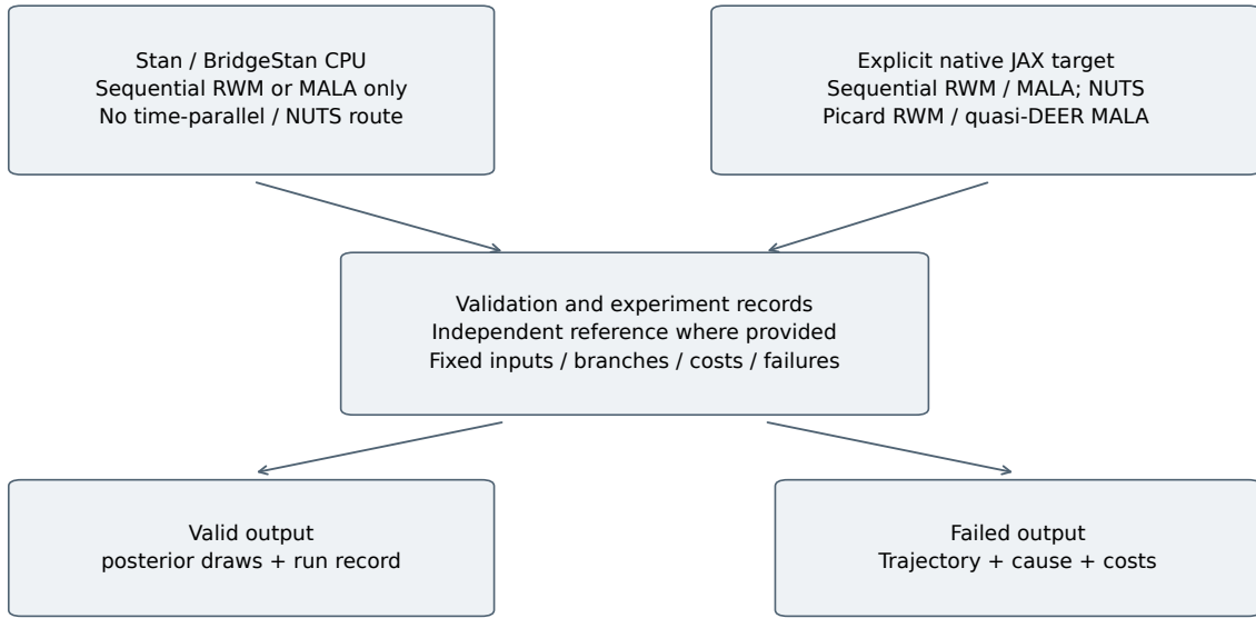
图 1: 计算与验证流程。目标、核和执行器分别记录，失败轨迹与正常后验对象分离。NUTS 使用自身随机流及预热过程，不继承固定噪声 MH 的轨迹比较。该图是程序逻辑示意，不含性能预测。
