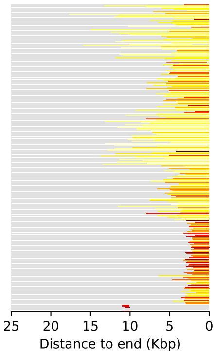
q-arm
