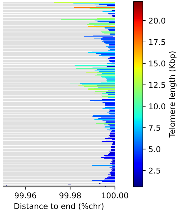
q-arm
