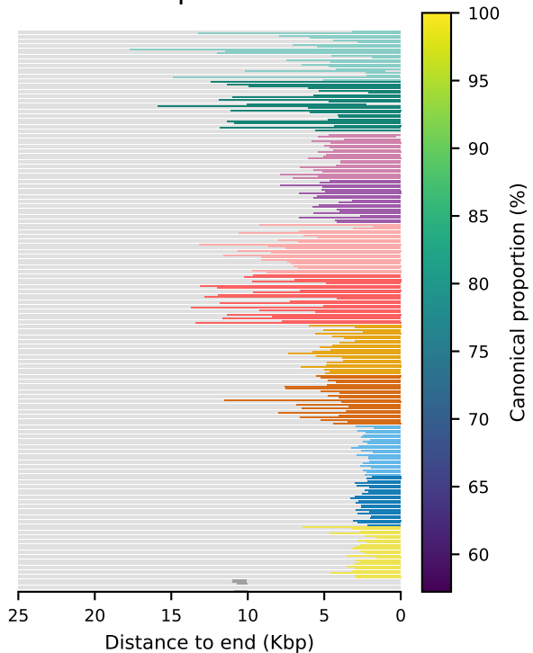
q-arm
