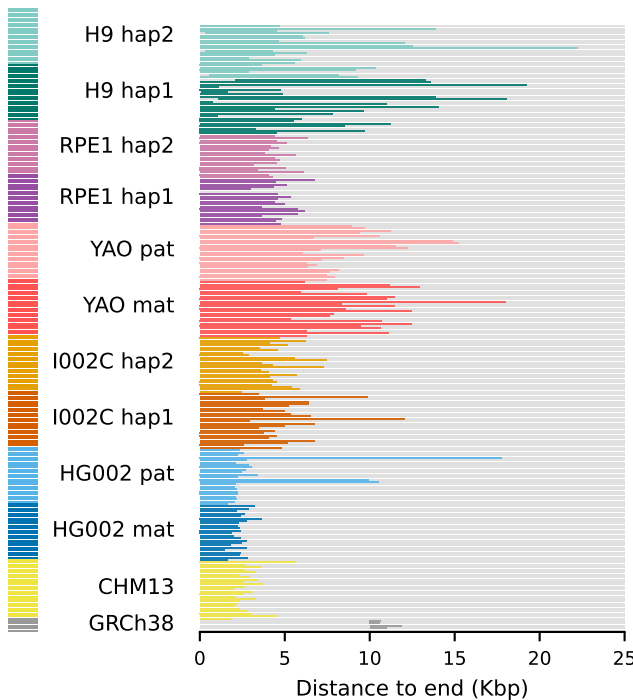
p-arm
