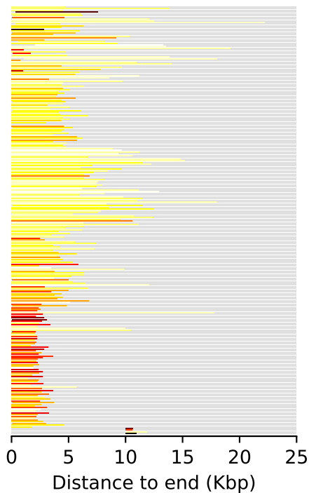
p-arm
