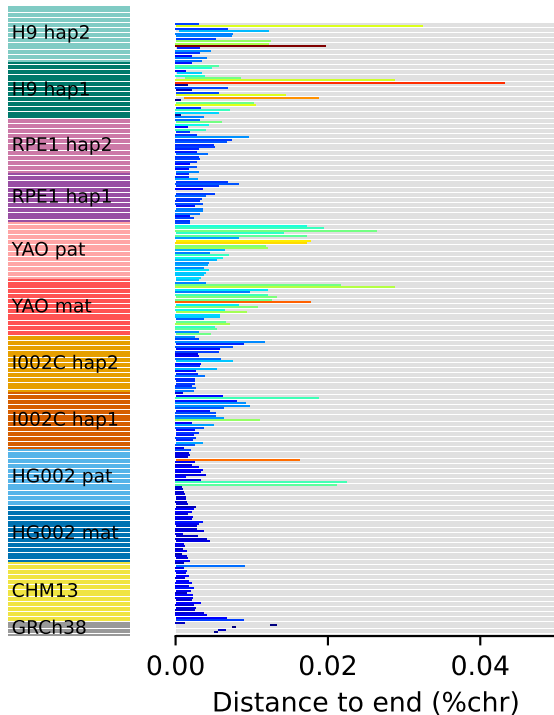
p-arm
