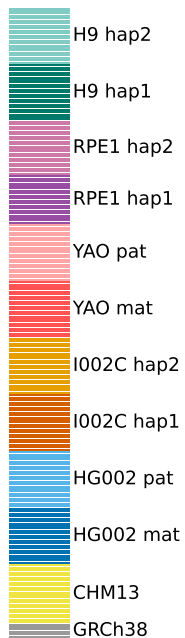
Telomere length (Kbp)
