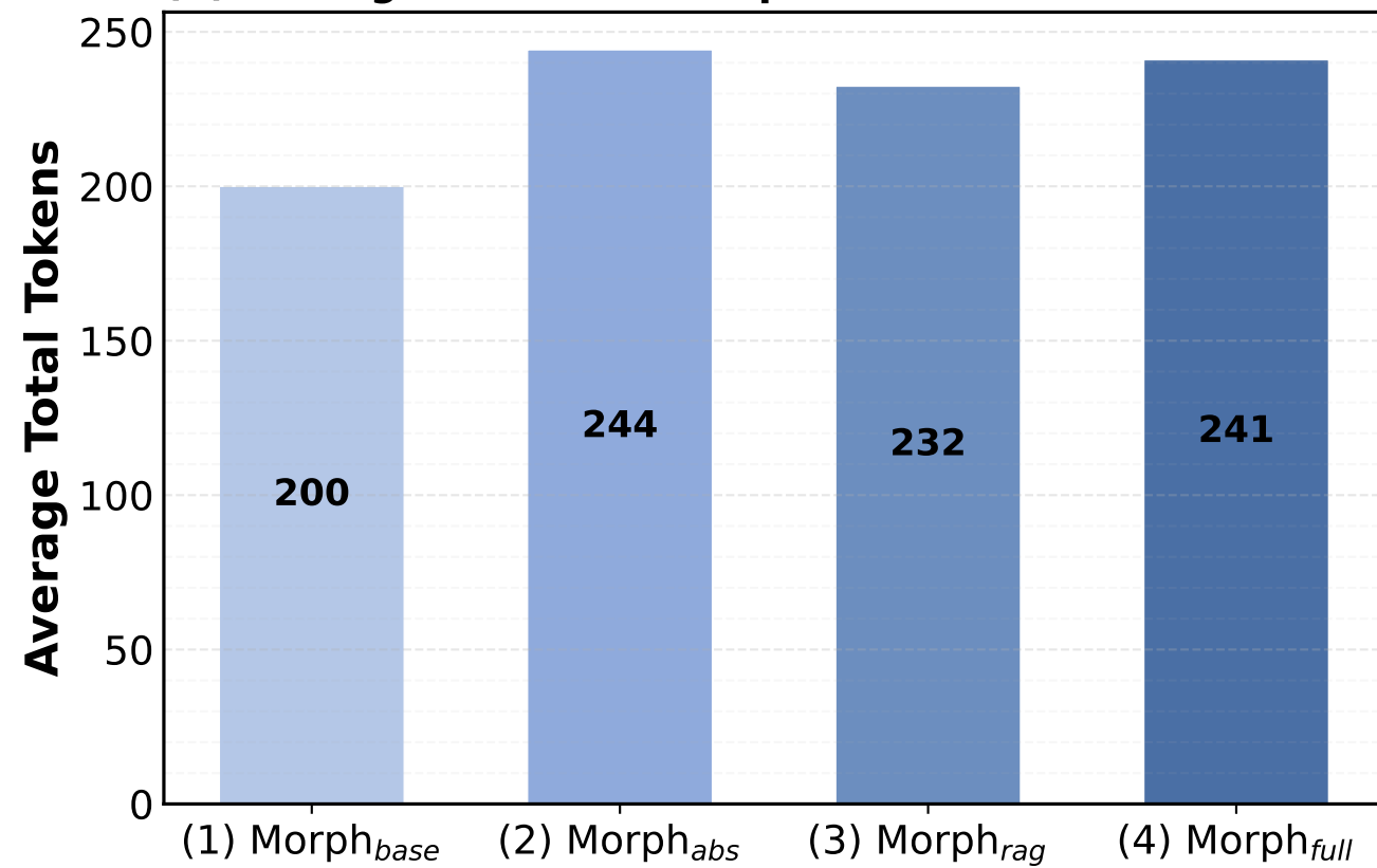
(d) Average Token Consumption
