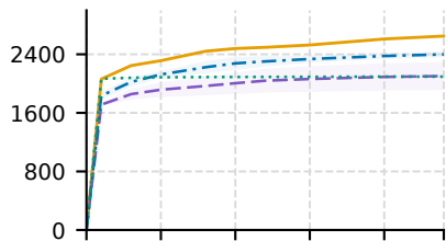
MySQL
