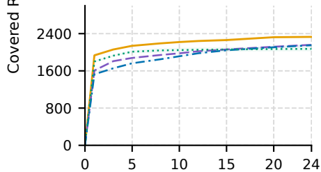
MariaDB
