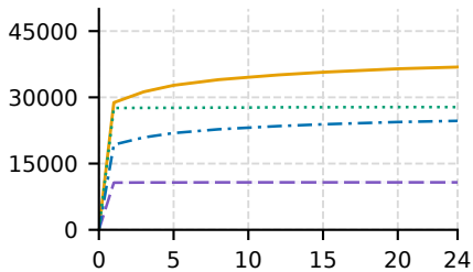
MonetDB
