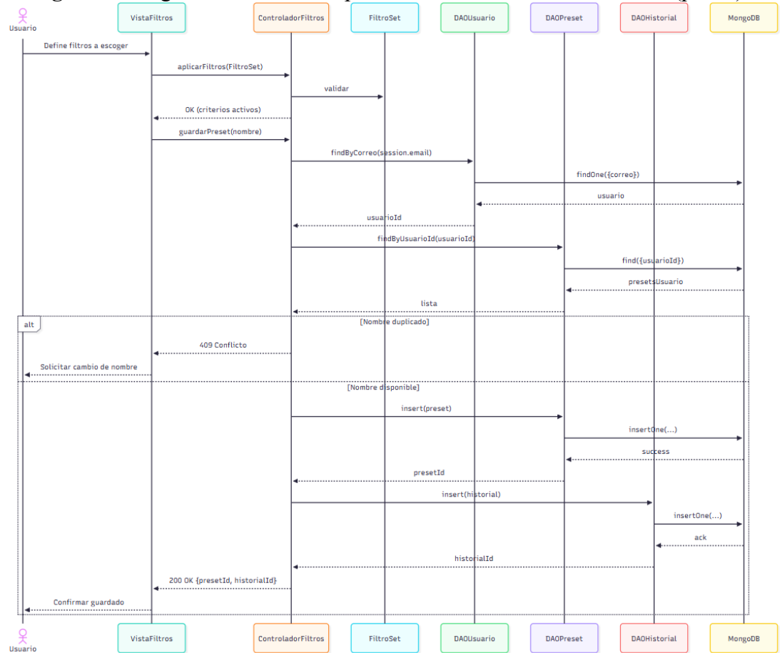
Figura 4: Diagrama de secuencia para el caso de uso “Guardar filtros (preset)”
