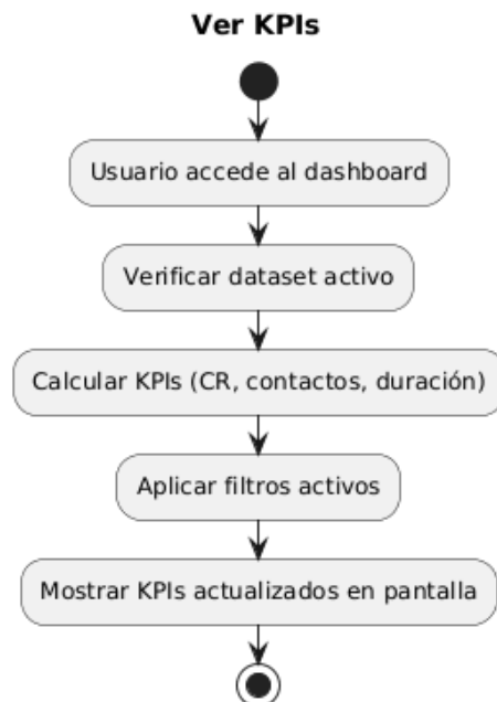
Figura 10: Diagrama de actividad de “Ver KPIs”
