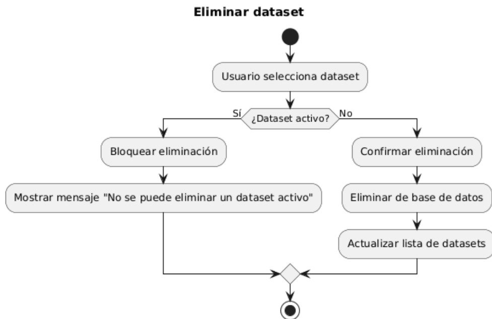
Figura 8: Diagrama de actividad de “Eliminar dataset”
