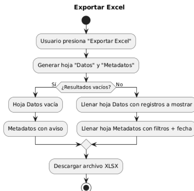
Figura 14: Diagrama de actividad de “Exportar Excel”
